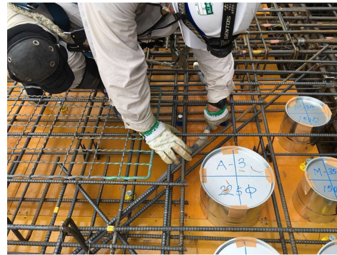
スラブ配管状況
