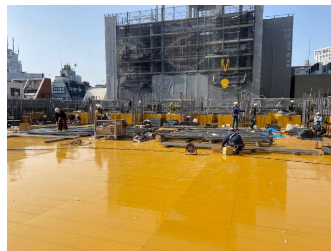
型枠組立状況
