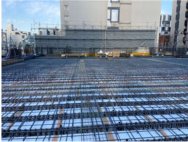
床配筋状況
