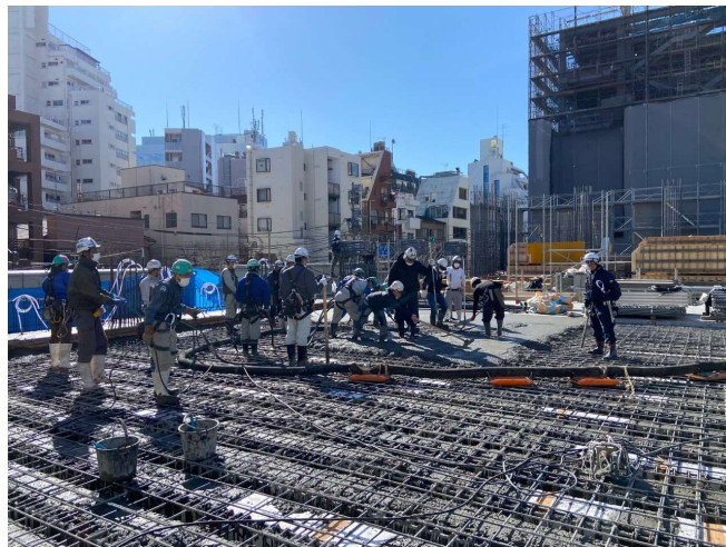
コンクリート打設②
