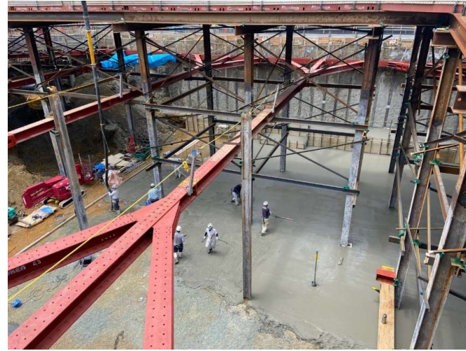
興風館コンクリート打設
