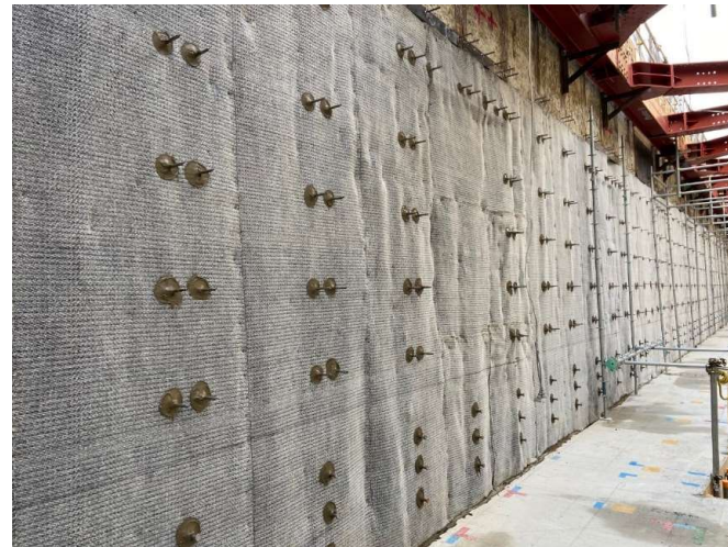
興風館地下外壁防水
