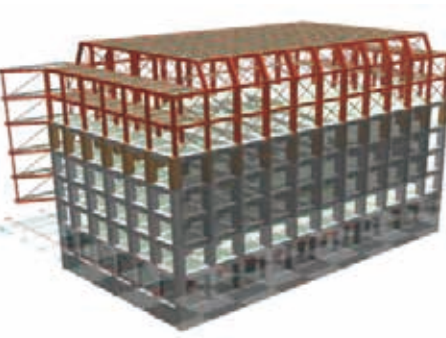
構造架構パース（興風館）
